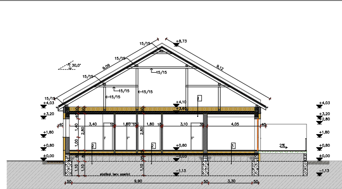
A-A METSZET
